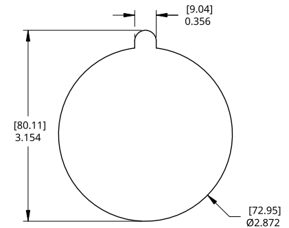
73 MM (2.87") TAB LID
